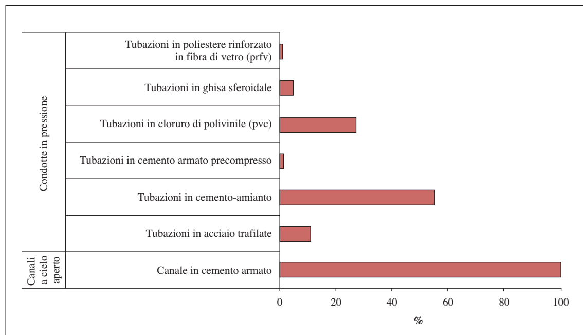
Grafico 4.7 - Principali materiali costituenti la rete
