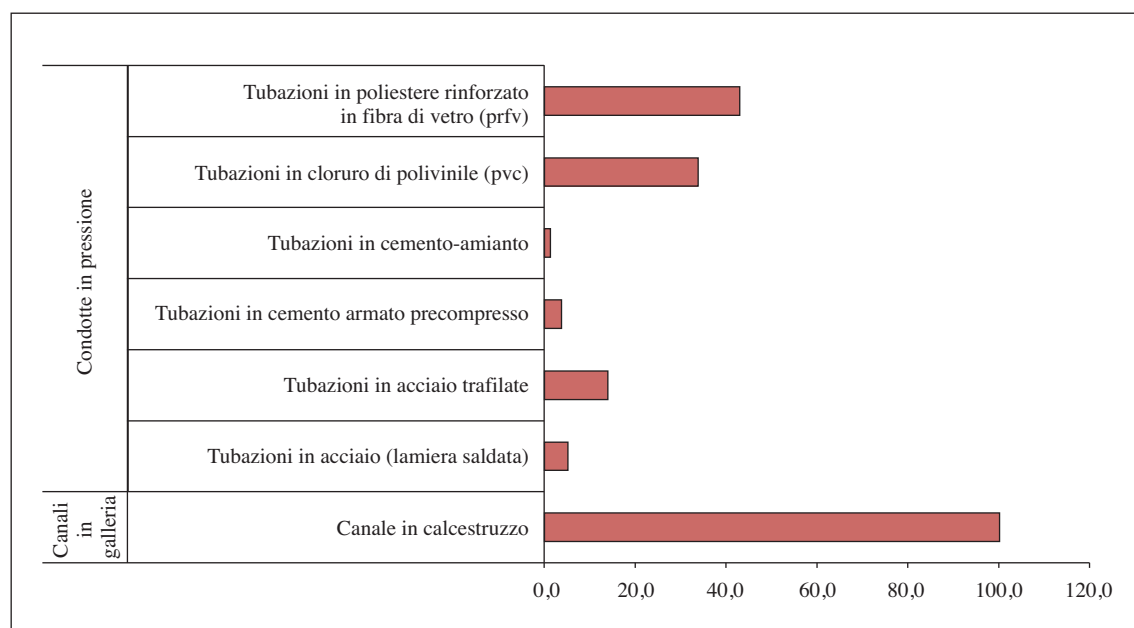
Grafico 4.6 - Schema irriguo Montedoglio - Materiali costruttivi della rete
